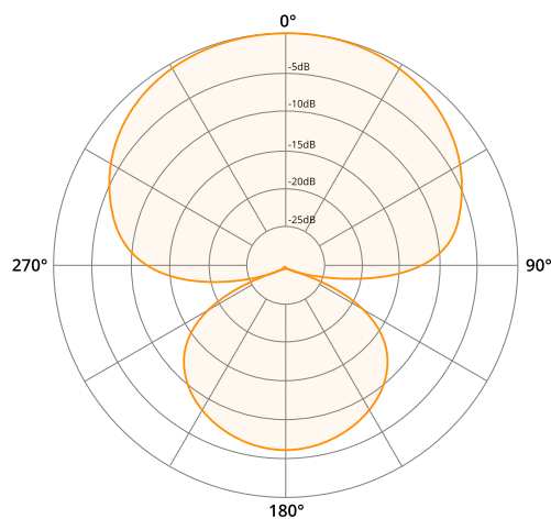
Hypercardioïde
