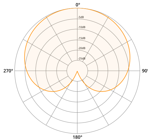
Cardioïde
