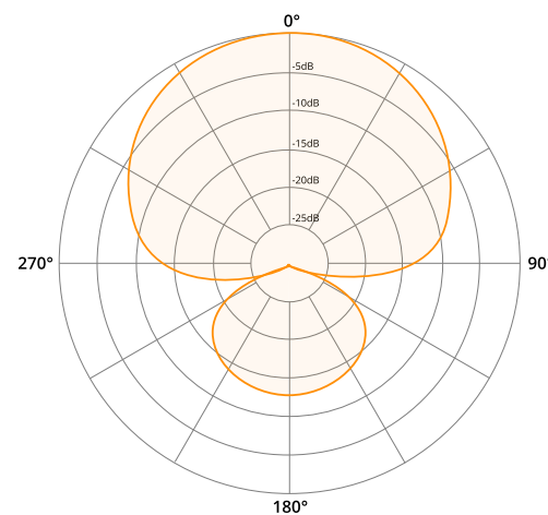
Supercardioïde
